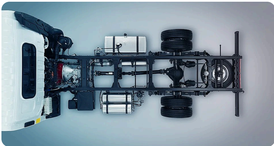
Chassi visto de cima: longarinas livres para o implemento
